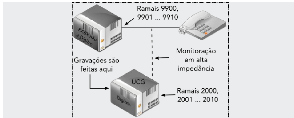
Figura 36. Exemplo de PABX legado e monitoração em alta impedância
