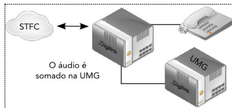
Figura 8. Gravação com soma na UMG
