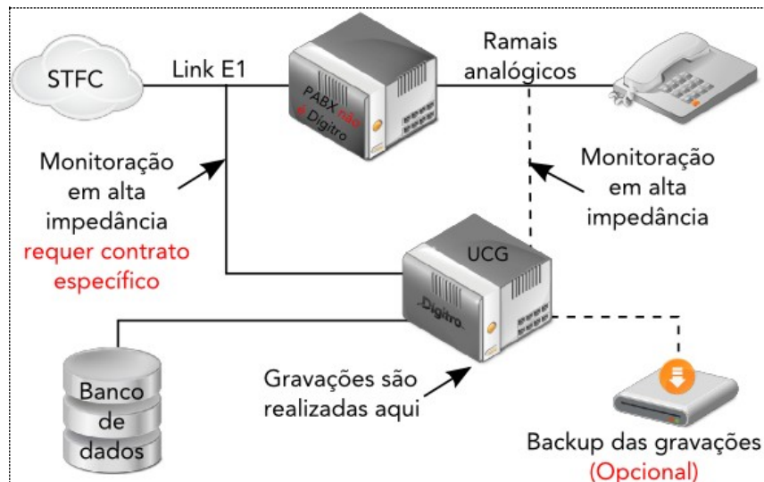
Figura 3. PABX em plataforma de terceiros + Gerenciamento e Gravação em plataforma Dígito
